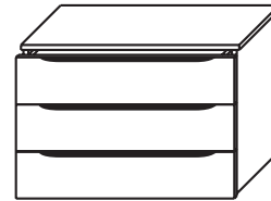
Schubkasteneinsatz, steingrau, 3 Schübe Maße: B/H/T 88/57/45 cm Art.-Nr. 499805
