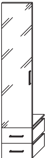
Spiegeltür, mit zwei Schubkästen und einem Konstruktionsboden Maße: B/H 45/221 cm
